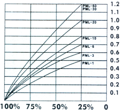
Luftspalt (mm)
