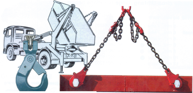
Kettengehänge mit Absetzkipperhaken und Verkürzerklaue mit Sicherung.
