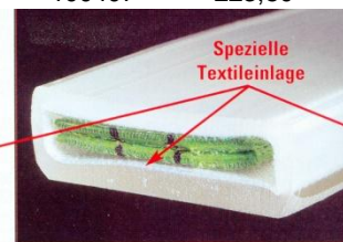
Profil - Schlauch mit zweiseitiger Beschichtung
